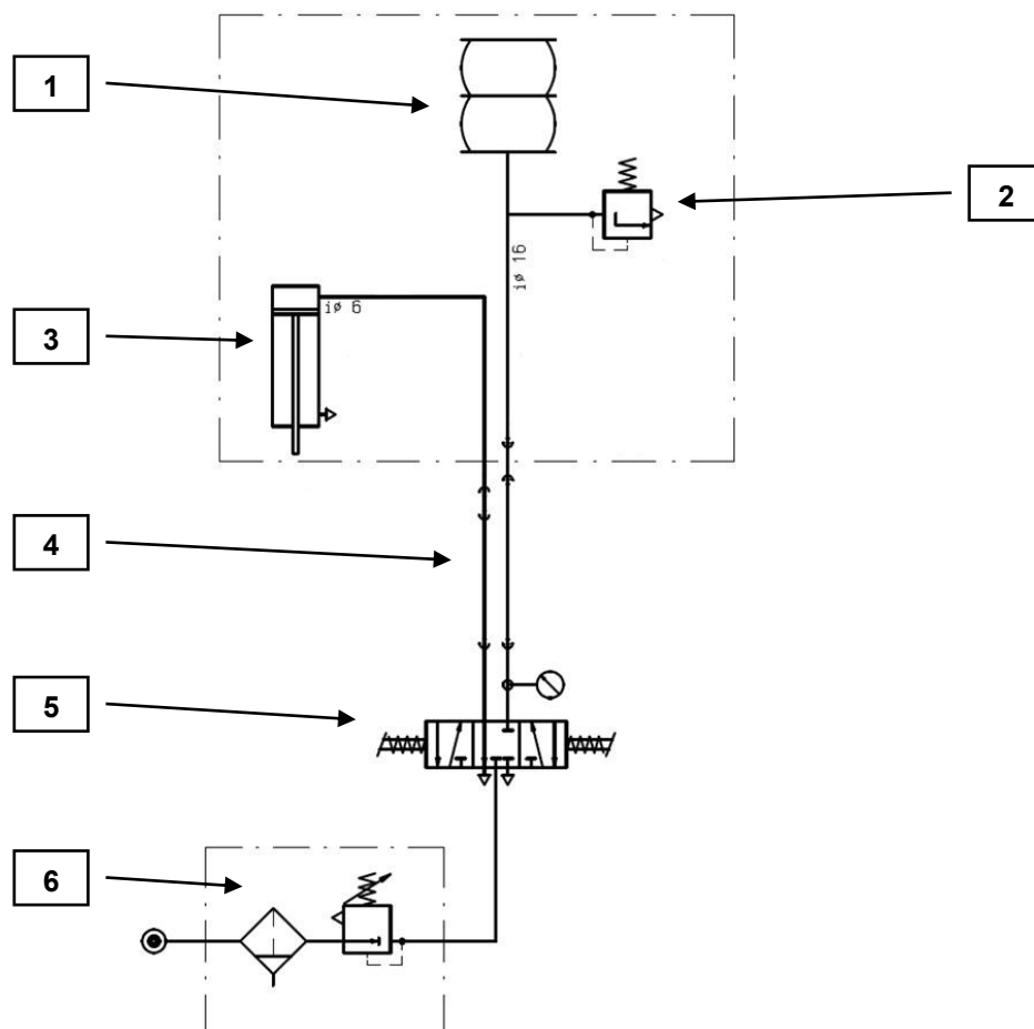
Bild 11: Pneumatikplan K1208
